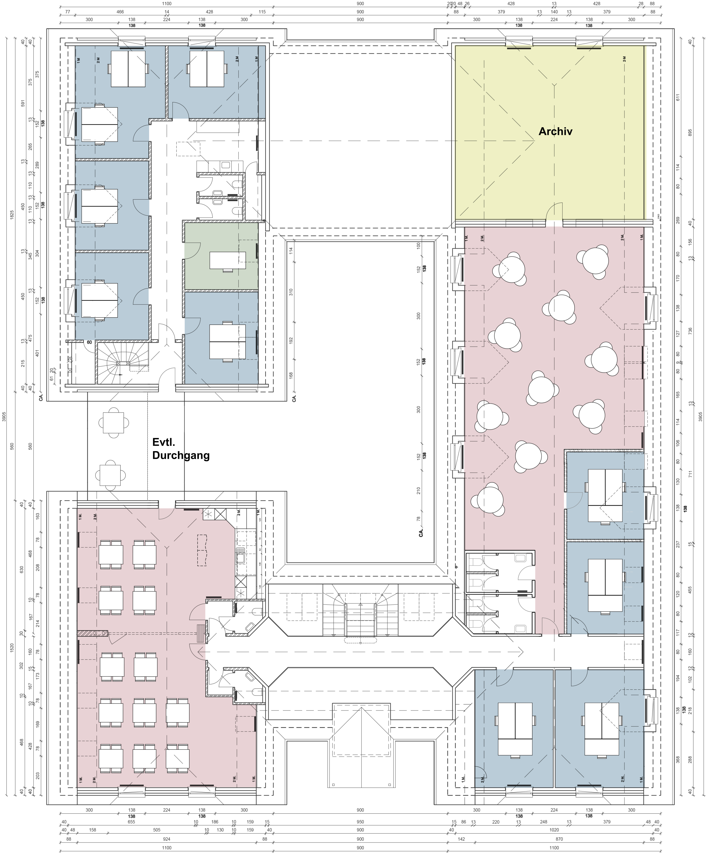
DACHGESCHOß 1:100
